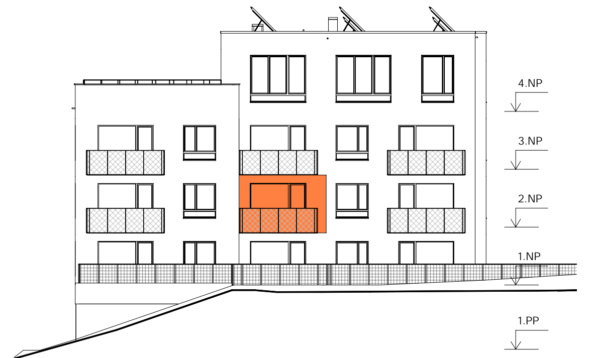
POHLED ZÁPADNÍ
