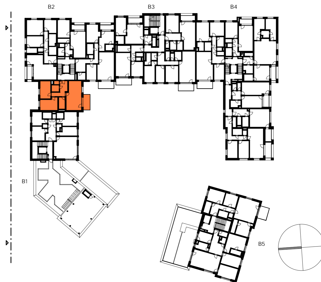
PŮDORYS 4.NP
